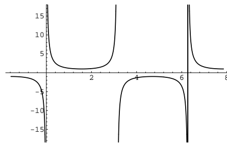
Figura 2.10: gráfica de cosec
