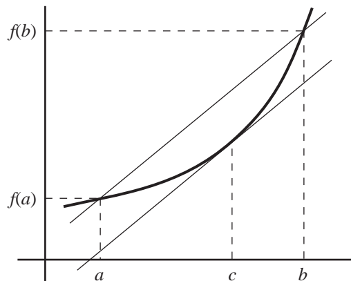
Figura 4.6: teorema del valor medio
