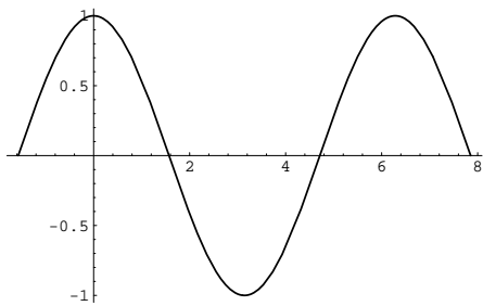
Figura 2.7: gráfica de cos
