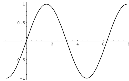
Figura 2.8: gráfica de sen
