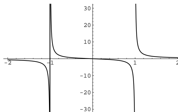
Figura 4.11: gráfica de la función f(x) = x/(x^2 - 1)
