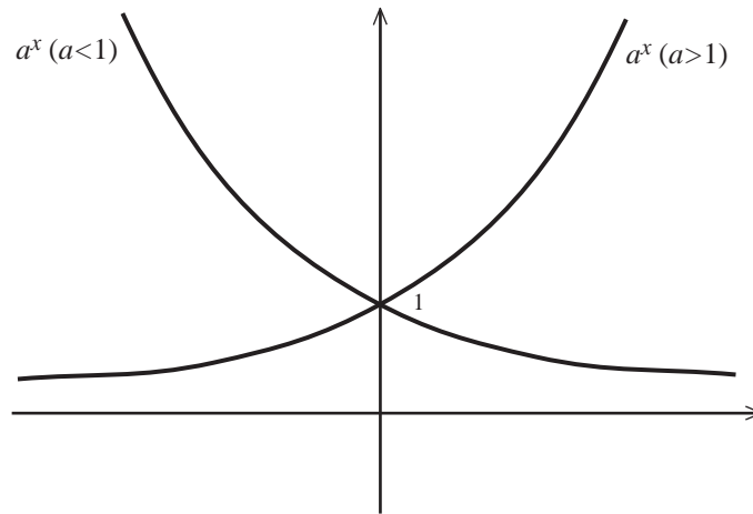
Figura 2.3: gráfica de la función a^x
