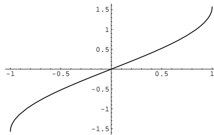
Figura 2.14: gráfica de arc sen
