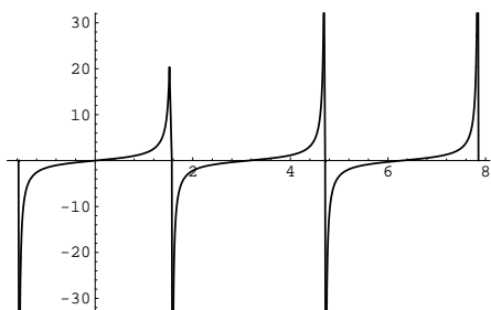
Figura 2.11: gráfica de tan
